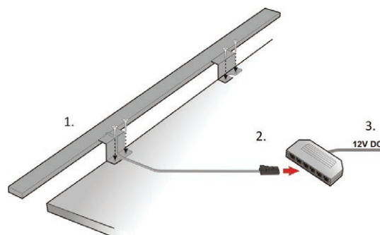
↑ schéma montáže a zapojenia na zrkadlá podlepené na ráme a zrkadlové skrinky
