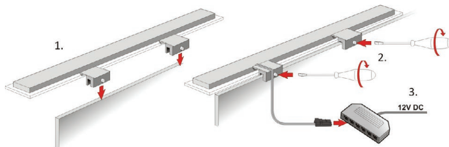
↑ schéma montáže a zapojenia na zrkadlá
